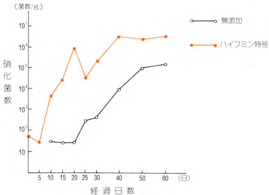
硝化能の推移(消毒殺菌)一園試土壤
