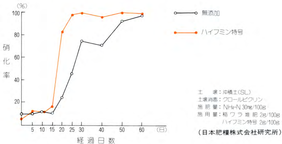
硝化能の推移(消毒殺菌)一園試土壤
